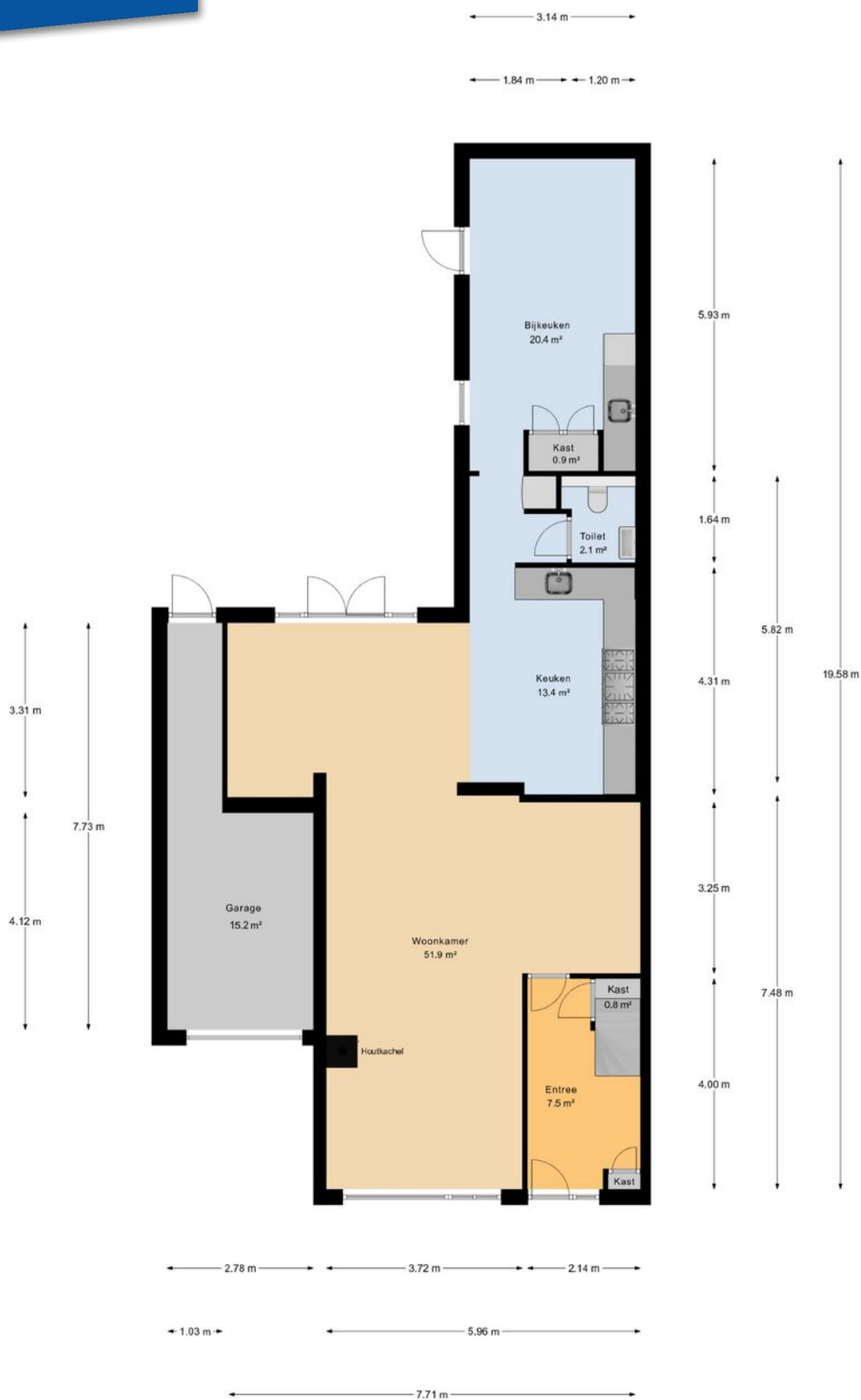
Begane Grond
